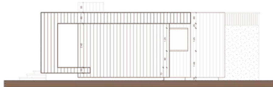
ELEVACIÓN SUR
